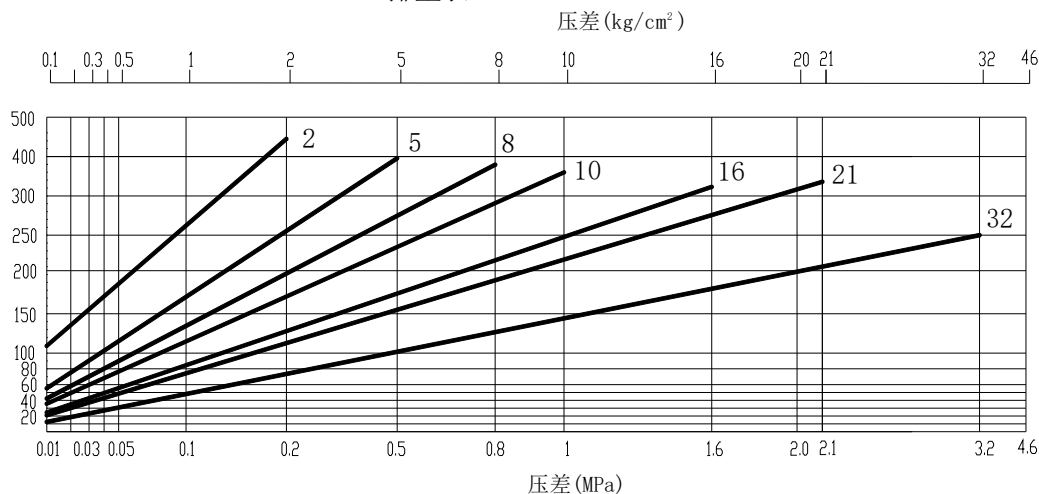
WY42S、WY42SU (DN15~DN25) 排量表
