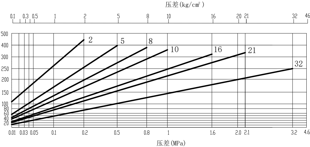
WY42F（DN15~DN25） 排量表
