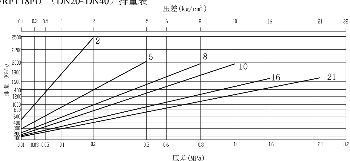
RFT18F /RFT18FU (DN20~DN40) 排量表
